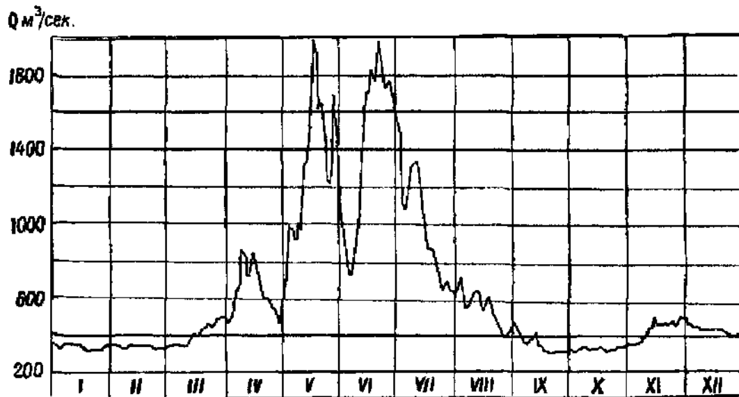
Рис. 2. Гидрограф реки Сырдарьи у г. Беговат за 1942 г. (Шульц, 1965)
