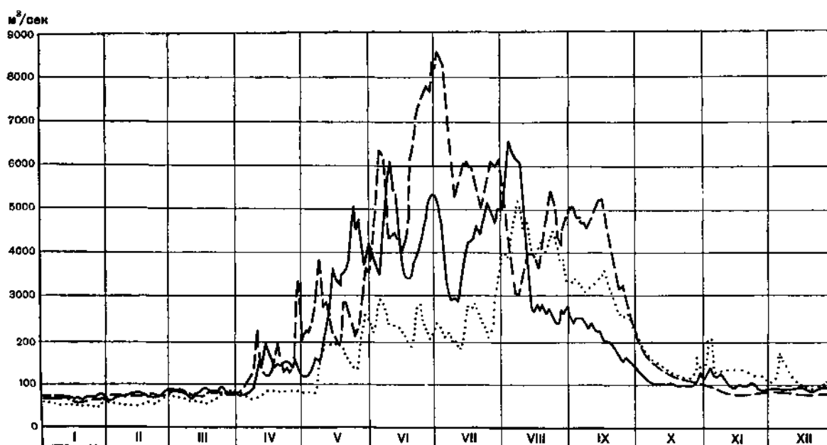
Рис. 1. Гидрограф реки Амударьи у г. Керки в годы разной водности, в \text{м}^3/\text{сек} (Соколов, 1964). Расходы воды: ----- 1914 г. максимум; ____ 1913 г. средний; ..... 1917 г. минимум
