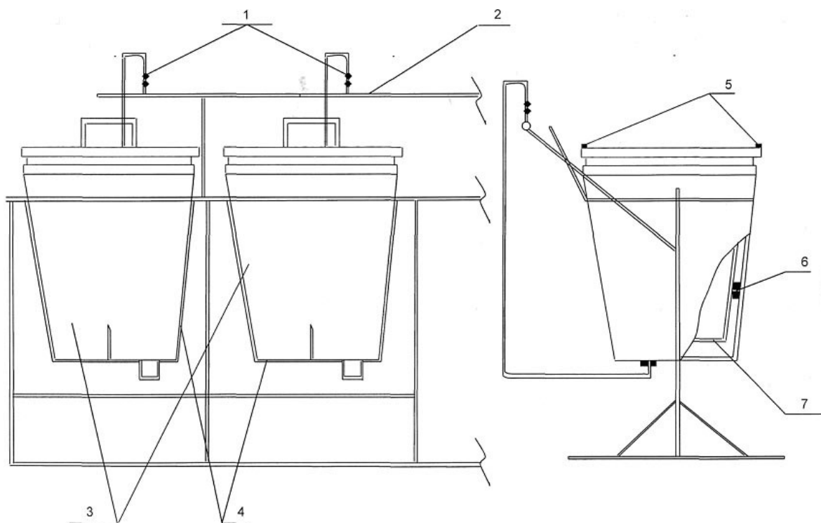
Рис. 4. Аппарат обесклеивания икры конструкции Шишкина Н.П. (АОИШ-1). 1 – вентили подачи воздуха; 2 – воздушная трубка; 3 – ведра для обесклеивания; 4 – корзина крепления ведер; 5 – саморезы (4 шт.); 6 – уплотнитель резина; 7 – перфорированное дно
