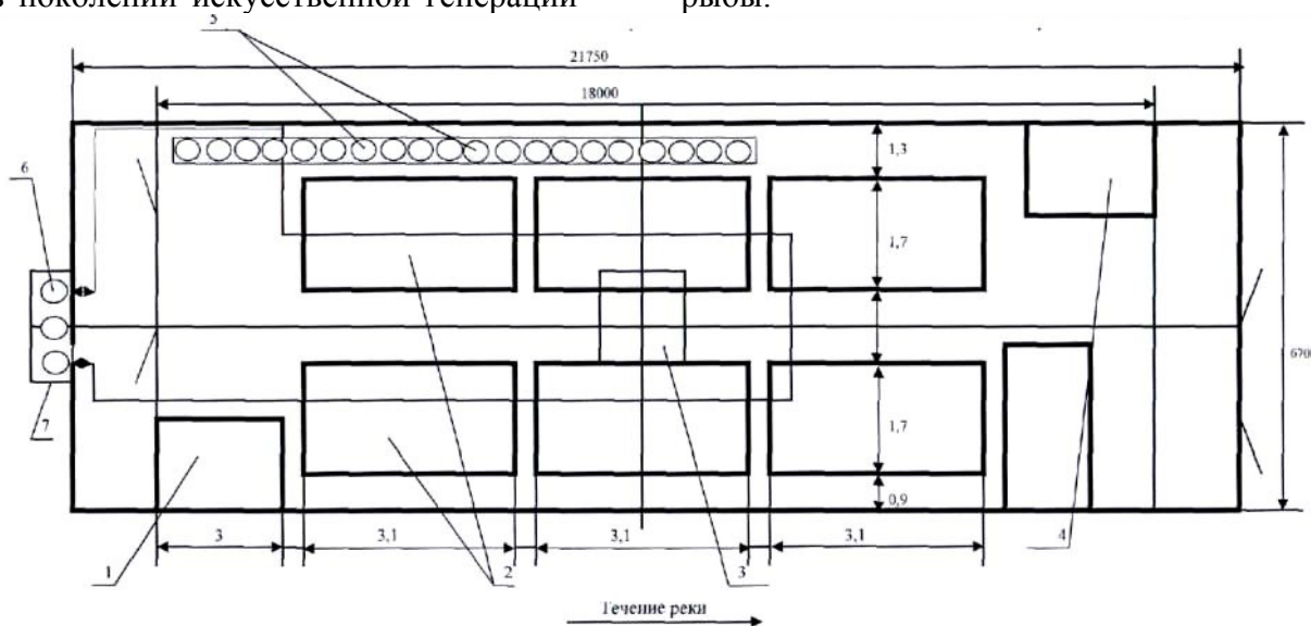
Рис. 2. Схема инкубационного цеха на понтоне. 1 – помещение лаборатории; 2 – инкубационные аппараты «Осетр»; 3 – ёмкость для раствора фиолетового «К»; 4 – помещение бытовки; 5 – аппараты для обесклеивания икры; 6 – насосы (3); 7 – рыбозащита
