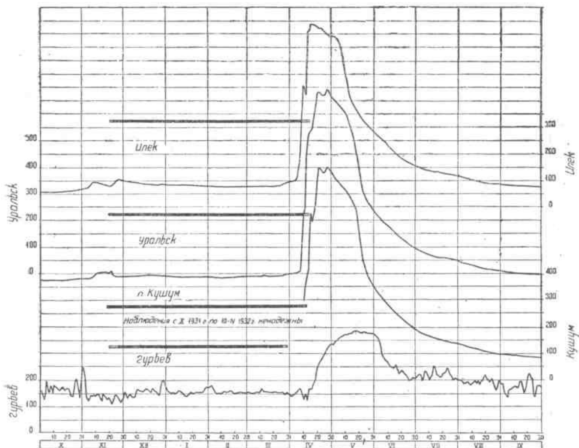
Рис. 4. Совмещенные графики уровней реки Урала от г. Илека до г. Гурьева (Атырау) за 1932 г., в см (Кокин, 1938)
