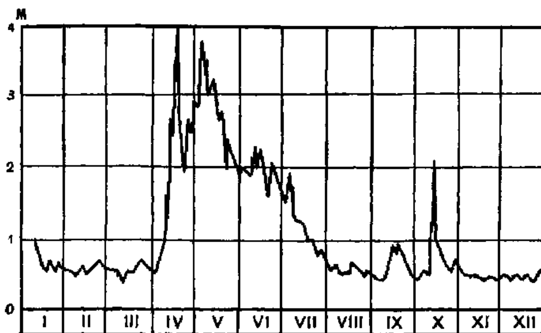
Рис. 5. Гидрограф реки Куры у с. Мингечаур за 1928 г., уровень в м (Соколов, 1952).
